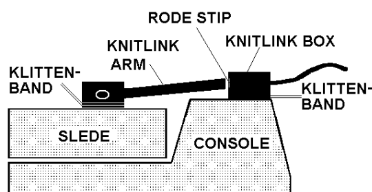
DesignaKnit USB link van opzij gezien
