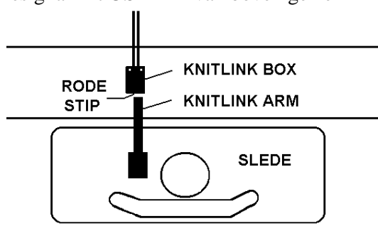
DesignaKnit USB link van boven gezien
